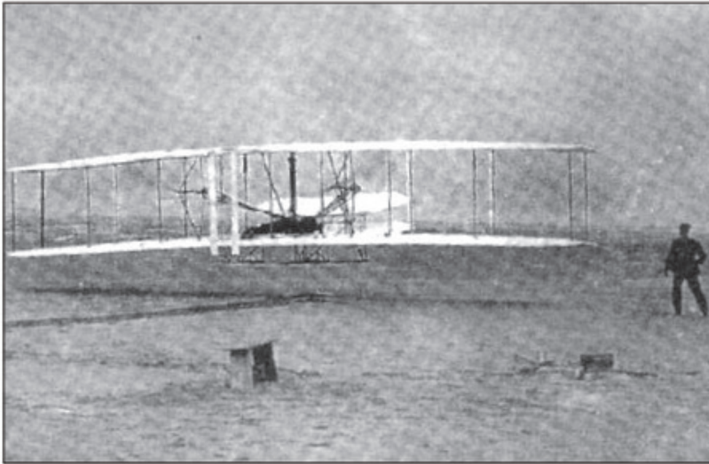
Hình 81. Chiếc máy bay đầu tiên trên thế giới (ngày 17 - 12 - 1903 bay được 12 giây) do hai anh em người Mĩ O-vin và Uyn-bơ Rai chế tạo
